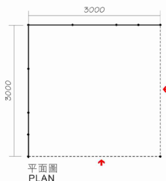
雙面入口攤位 Two Side Open
