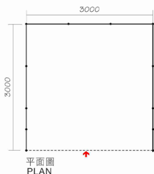
單面入口攤位 One Side Open
